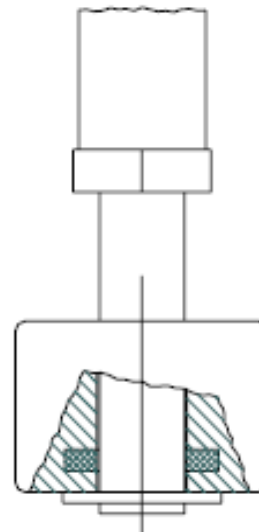
CONNEXION ÉLECTRIQUE NIVEAU CONTACT OUVERT QUAND LE RESERVOIR EST VIDE
