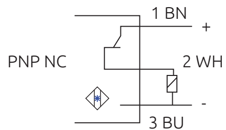
Schaltplan
